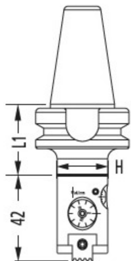
Disco de Graduação
